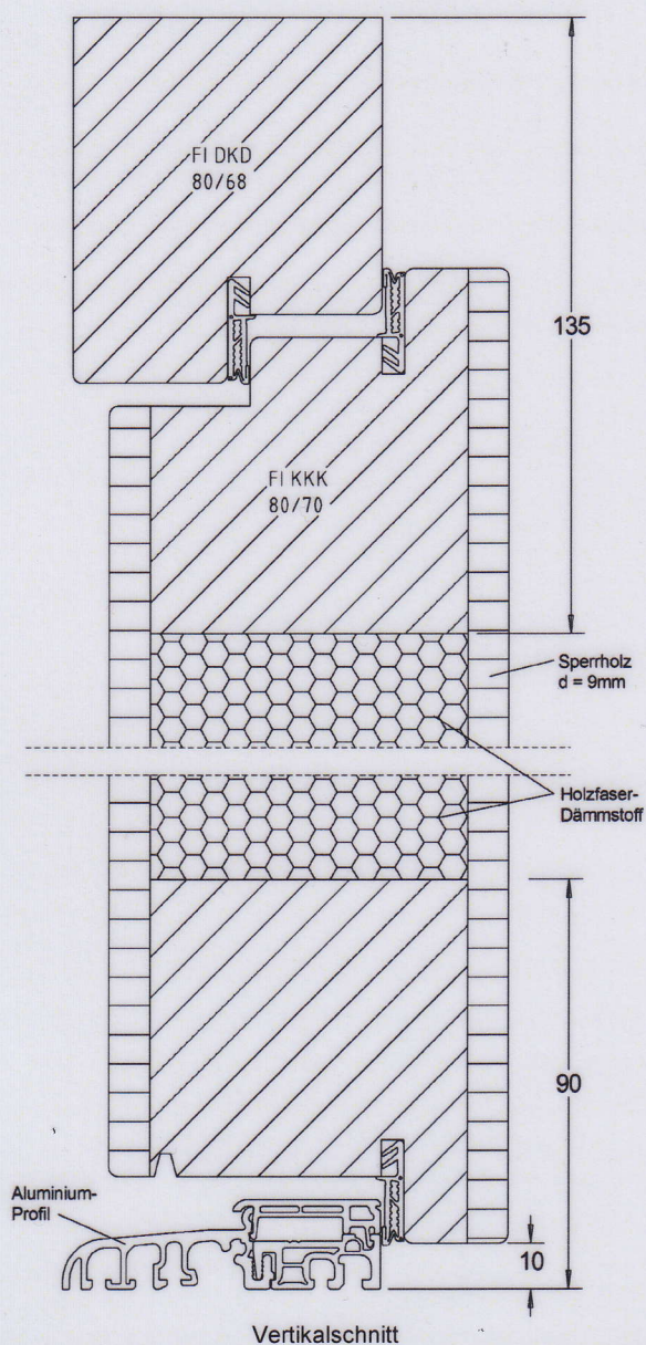
Vertikalschnitt
