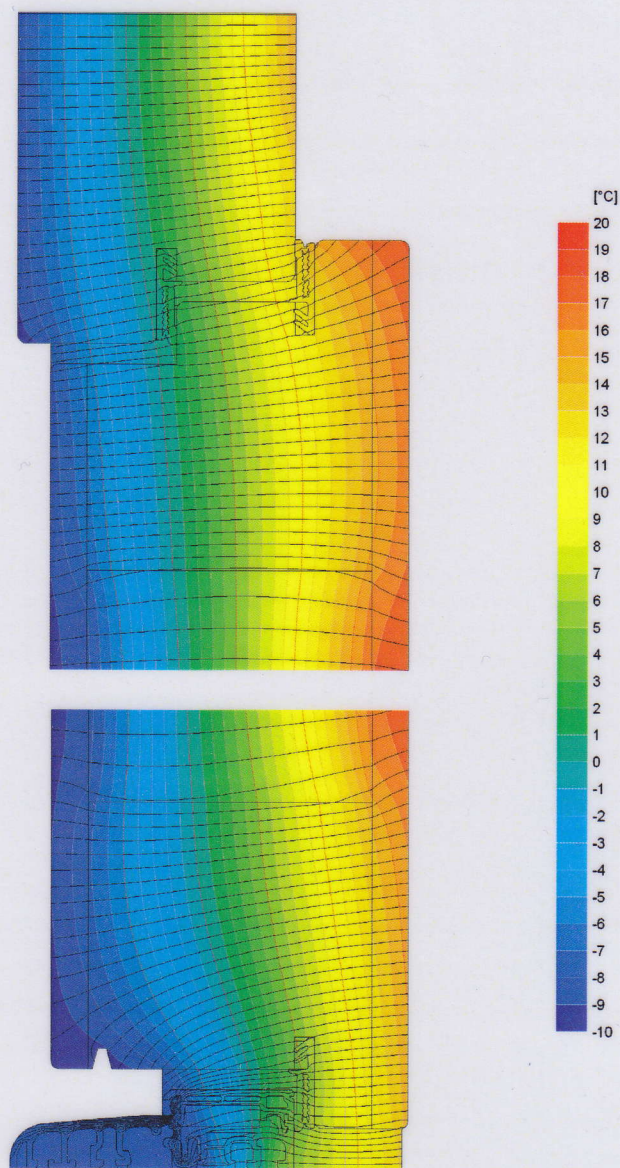
Isothermen- und Wärmestrombild
